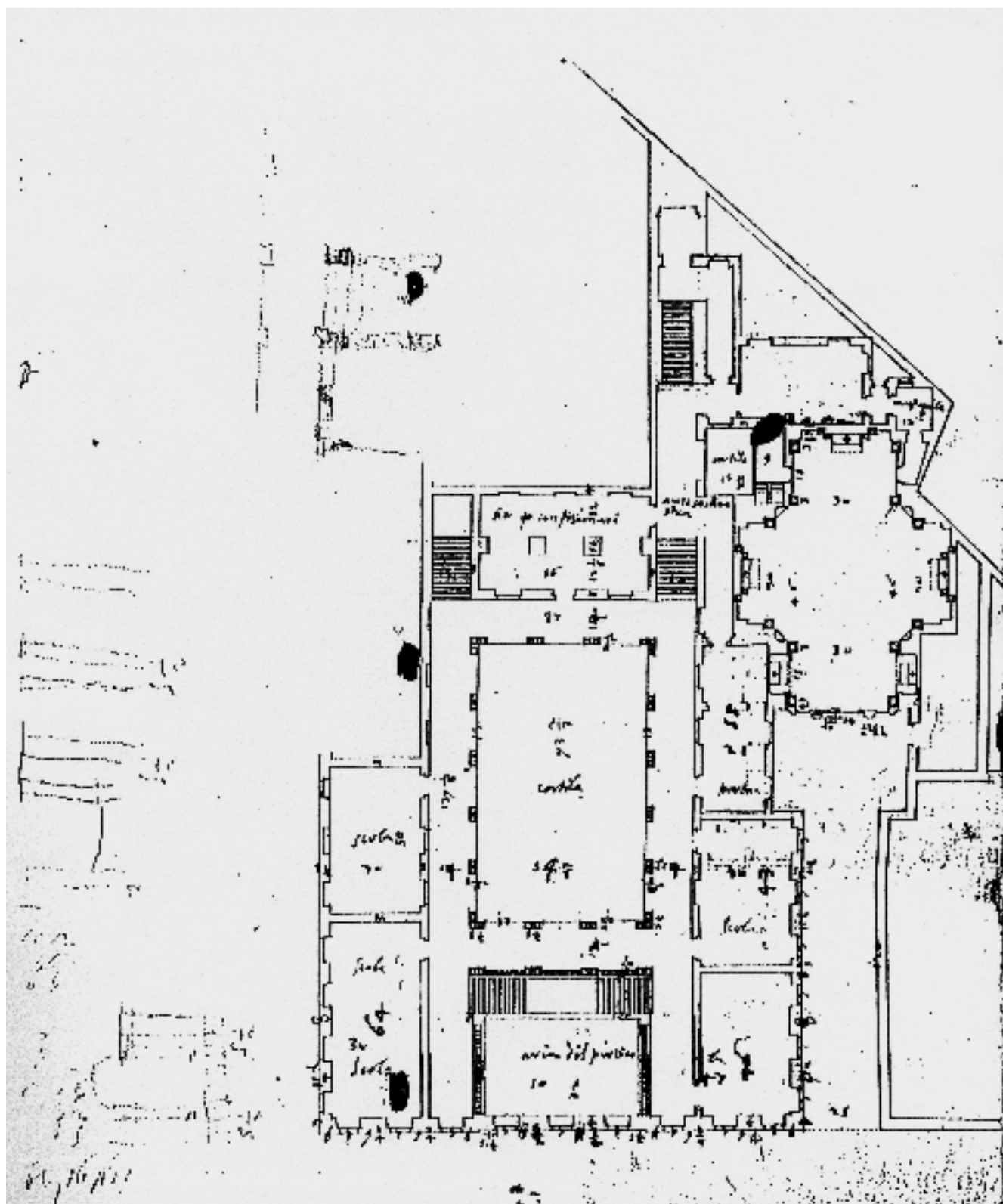
102. Genua, Kolleg, Plan Nr. 10, Gesamtentwurf, Grundriss der Kirche und des Schulgebäudes.
